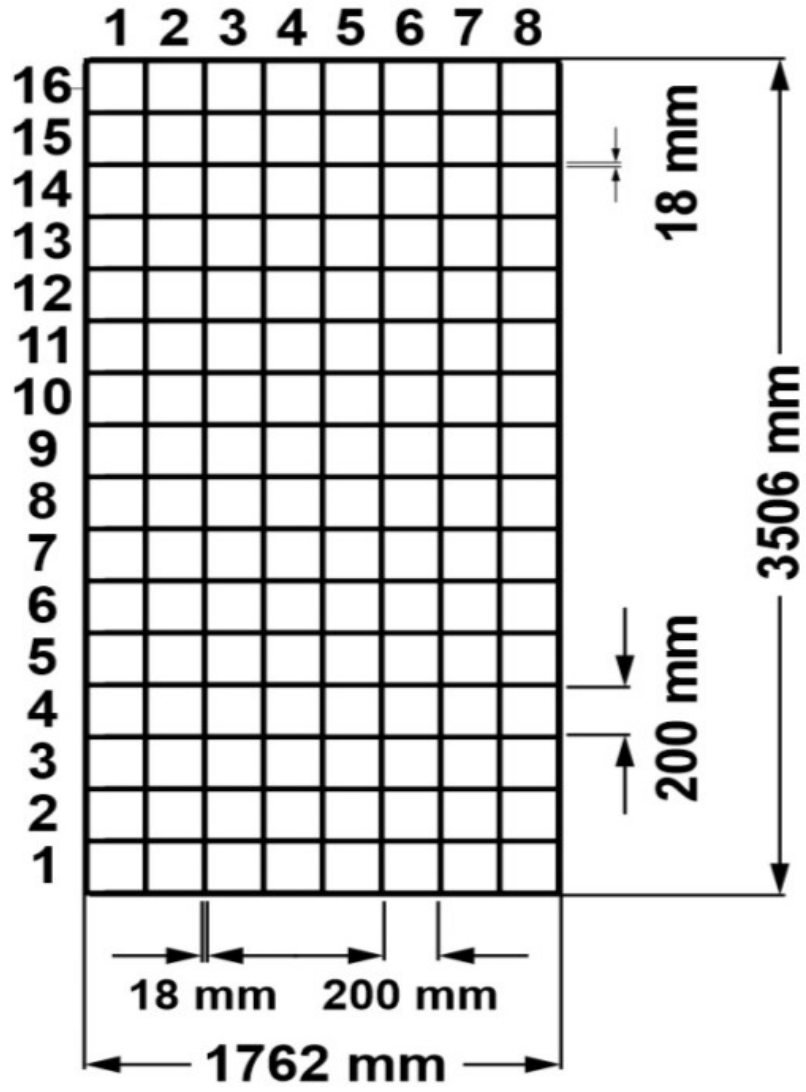
Şekil 4. Pist Ölçüleri
